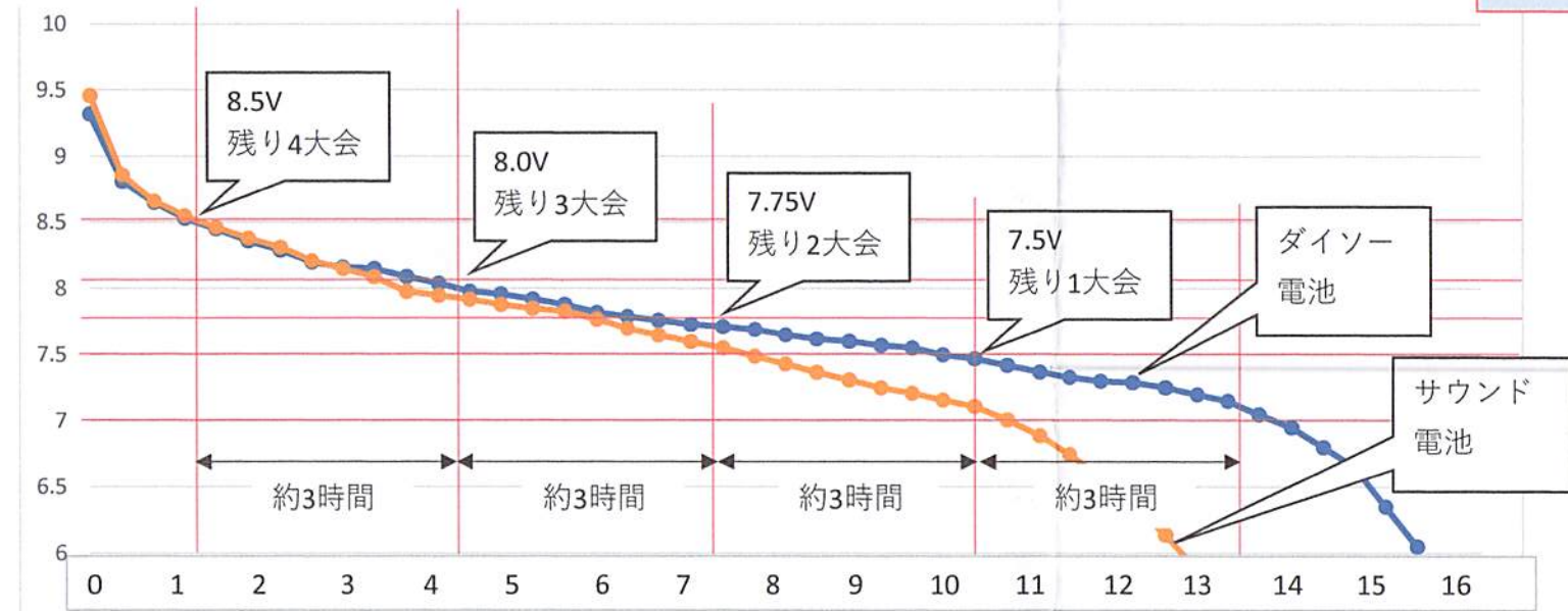
電池電圧 006P容量チェック (負荷30mA)
