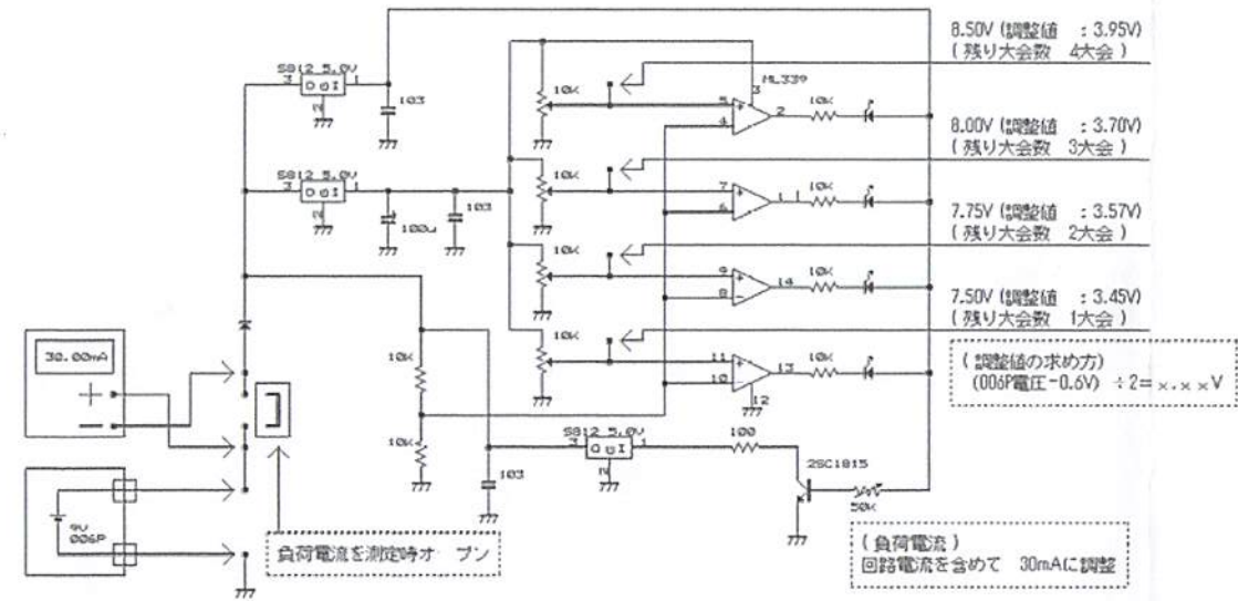
電池電圧 006P容量チェック (負荷30mA)
